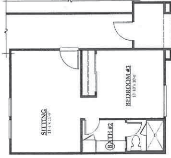
CASITAS OPTION
